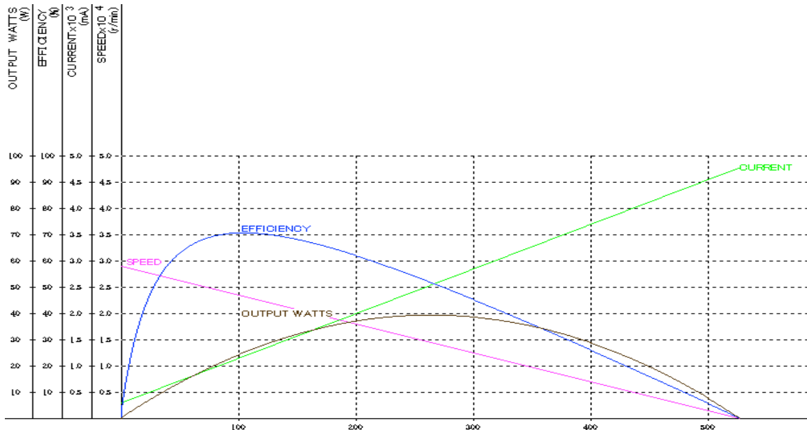
特性図 (Characteristics)
