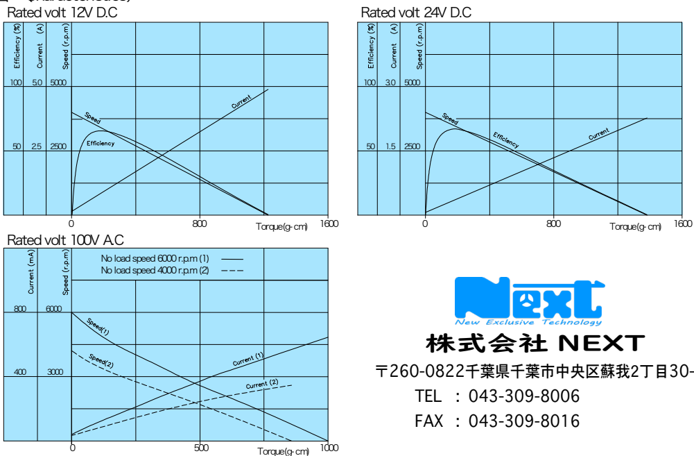
特性図 (Characteristics)
